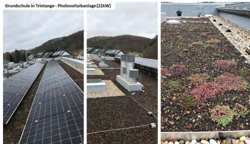
Grundschule in Trintange - Photovoltaikanlage (22kW)
